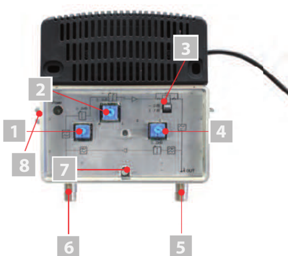
Bild 2: Verstärker HVB 31, Innenansicht
